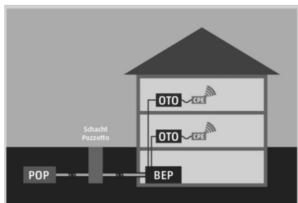
Schema collegamenti
