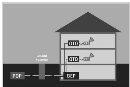
Verteilerschema
